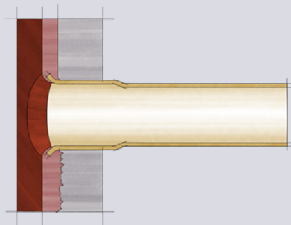
plastocor® 覆层系统 用于管板保护
