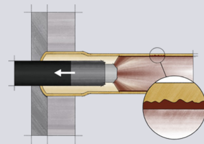
plastocor® 管道内衬系统 用于全长管道保护
