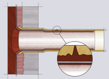
Sistema plastocor ® Inlet para protección de entrada/salida de tubos
