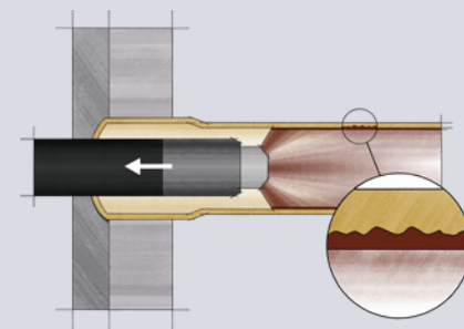
Sistema plastocor ® Tube Lining para protección de toda la longitud del tubo
