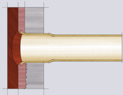
Sistema plastocor ® Cladding para protección de placa tubular
