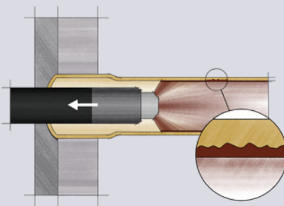
plastocor® Система покрытия для защиты внутренней поверхности трубок по всей длине
