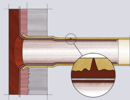
plastocor® Система покрытия для защиты входных и выходных участков трубок
